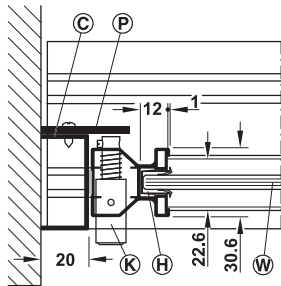
Lock on wall connection profile วิธีการติดตั้งโปรไฟล์เชื่อมต่อผนัง
