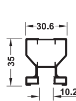
Lateral frame profile No.10 เฟรมด้านข้างเบอร์ 10
