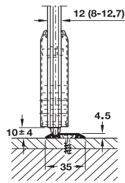
Built-in version 1 โก๊ตส์ล่าง รูปแบบที่ 1
