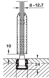
Built-in version 2 โก๊ตส์ล่าง รูปแบบที่ 2
