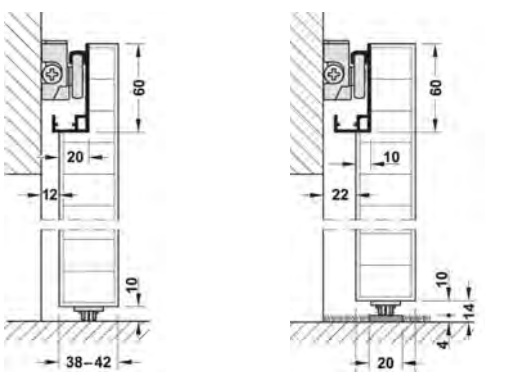
Floor guide on hard floor การติดตั้งแบบกันแกว้งใต้บาน
