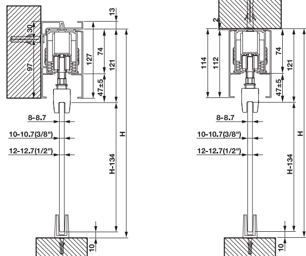
Wall installation with glass panel ติดตั้งบนผนัง สำหรับประตูบานกระจก
