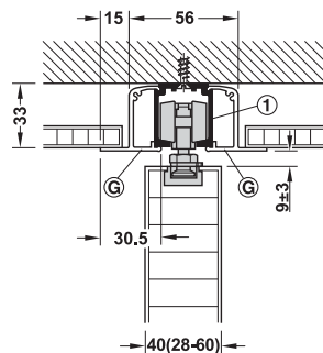
Ceiling installation with running track and 2 x clip panel for integration in suspended ceilings การติดตั้งบนเพดานด้วยรางและฝาครอบพร้อมแผ่นปิดด้านล่าง 2 ชิ้น
