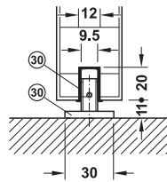
With guide track แบบติดตั้งรางได้บาน
