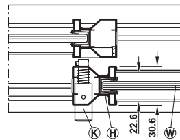
Lock on rear door วิธีติดตั้งเข้ากับบานประตู
