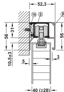
Wall mounting with running track, mounting rail high, width 8 mm, and clip panel 56 mm การติดตั้งบนผนังด้วยรางยึดผนังกว้าง 8 มม. และฝาครอบรางแบบคลิก 56 มม.
