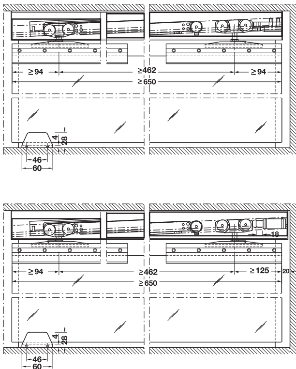
Wall installation with glass panel ติดตั้งบนผนัง สำหรับประตูบานกระจก
