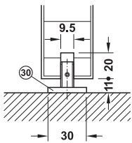
Without guide track แบบไม่มีรางได้บาน
