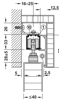
Wall mounting with mounting bracket and fixing clip for wooden panel การติดตั้งบนผนังด้วยเพลาติดผนัง และฝาปิดแบบคลิกสำหรับบานไม้
