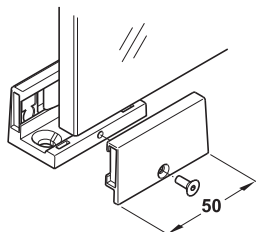
Wall profile set include rubber seal การติดตั้งรางที่ผนัง
