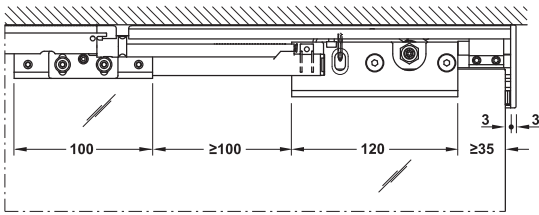
Section trolley hanger 40–50 kg with soft closing mechanism ระยะการติดตั้งสำหรับแขนลูกล้อ 40-50 กก.
