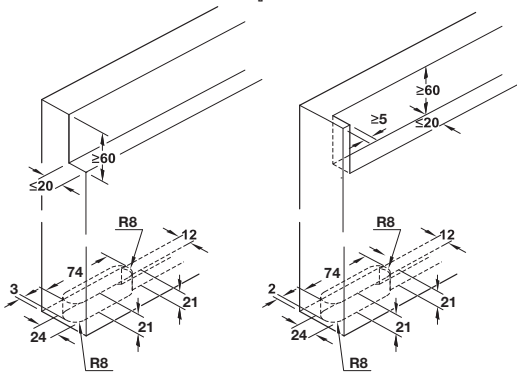
With end cap แบบฝาปิดปลายราง
