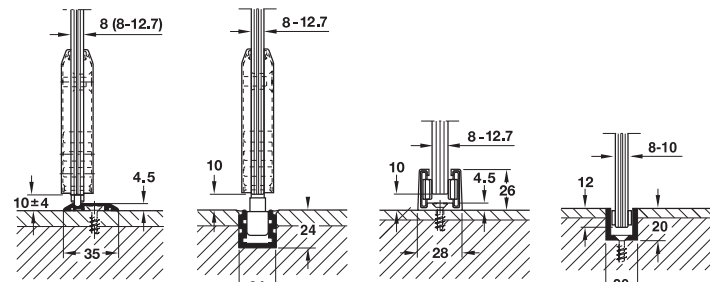
Built-in version 1 Built-in version 2 Built-in version 3 Built-in version 4 โกดกลาง รูปแบบที่ 1 โกดกลาง รูปแบบที่ 2 โกดกลาง รูปแบบที่ 3 โกดกลาง รูปแบบที่ 4
