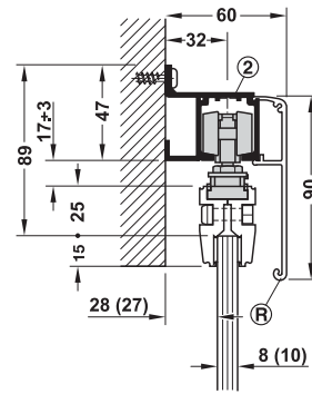
Wall mounting with running track and clip panel 90 mm การติดตั้งรางบนผนังและฝาครอบราง แบบคลิก 90 มม.
