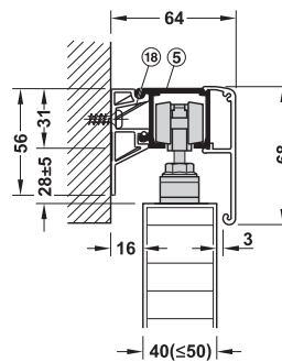
Wall mounting with running track, mounting rail high, width 19 mm, and clip panel 68 mm การติดตั้งบนผนังด้วยรางยึดผนังกว้าง 19 มม. และฝาครอบรางแบบคลิก 68 มม.
