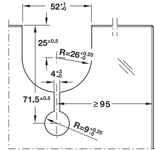
Required glass cut-outs กรุณาตัดกระจกตามรูปแบบที่กำหนดเท่านั้น
