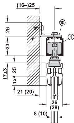
Wall mounting with wall mounting bracket ติดตั้งบนผนังด้วยเหล็กจากติดตั้ง
