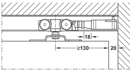
Track stopper with magnetic pull อุปกรณ์หยุดบานผลึกเพื่อเปิดแบบมีแม่เหล็ก
