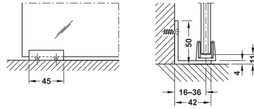
Section floor guide ระยะการติดตั้งสำหรับอุปกรณ์กันแกว่ง
