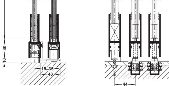
Telescopic without fixed panel การติดตั้งแบบไม่มีบานตาย
