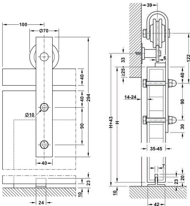
Section trolley hanger and guide ระยะติดตั้งลูกล้อและกันแกว่งบาน
