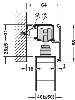
Wall mounting with running track, mounting rail, width 19 mm, and clip panel 68 mm การติดตั้งบนผนังด้วยรางยึดผนังกว้าง 19 มม. และฝาครอบรางแบบคลิก 68 มม.
