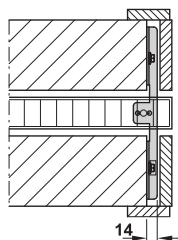
Floor guide, for wall mounting, with zero clearance กันแกว่งสำหรับบานซ่อนผนัง
