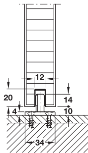
With guide track แบบติดตั้งรางล่าง
