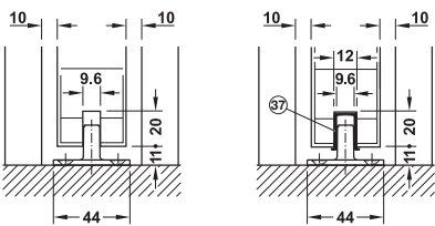
Without guide track แบบไม่มีรางใต้บาน
