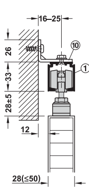
Wall mounting with mounting bracket การติดตั้งบนผนังด้วยเหล็กจากติดผนัง
