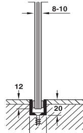
Built-in version 3 โก๊ตส์ล่าง รูปแบบที่ 3
