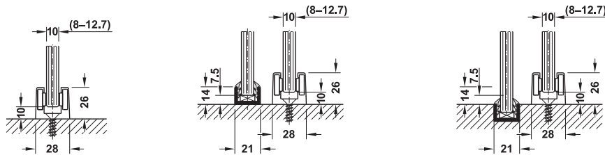
Floor guide ติดตั้งโดยกันแกว่งบาน
