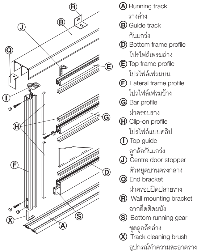
Lateral frame profile 20 เฟรมด้านข้างเบอร์ 20
