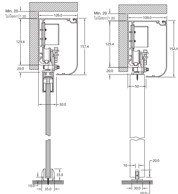
Glass frameless doors 12 mm ประตูกระจกเปลือย 12 มม.
