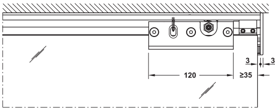
Section trolley hanger 40–50 kg ระยะการติดตั้งสำหรับแขนลูกล้อ 40-50 กก.
