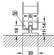
Floor guide กันแกว่ง
