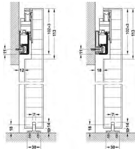
Wall distance 12 mm model A1, E1 ระยะห่างระหว่างบานประตูและผนัง 12 มม. รูปแบบ A1, E1
