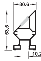
Lateral frame profile No.10-C Only for use in combination with lateral frame profile No.10, for 90° corner solutions เฟรมด้านข้างเบอร์ 10-C ใช้กับเฟรมเบอร์ 10 สำหรับติดตั้งแบบ 90°
