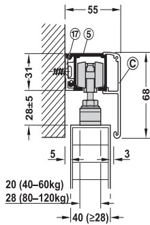
Wall mounting with running track, mounting rail, width 8 mm, and clip panel 68 mm การติดตั้งบนผนังด้วยรางยึดผนังกว้าง 8 มม. และฝาครอบรางแบบคลิก 68 มม.
