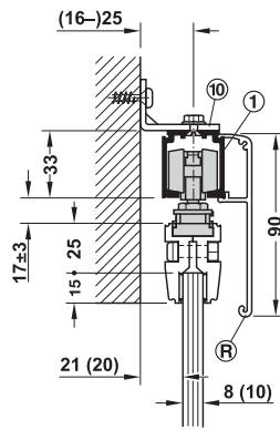
Wall mounting with wall mounting bracket and clip panel 90 mm การติดตั้งบนผนังด้วยเหล็กจากติดตั้ง และฝาครอบรางแบบคลิก 90 มม.
