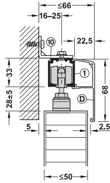
Wall mounting with concealed mounting bracket and wide clip panel 68 mm การติดตั้งบนผนังด้วยเหล็กจากติดผนัง และฝาครอบรางแบบคลิก 68 มม.
