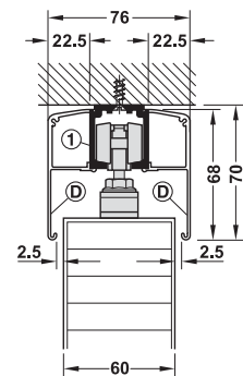
Ceiling installation with running track and 2 x wide clip panel 68 mm การติดตั้งบนเพดานด้วยรางและฝาปิดแบบคลิก 68 มม. 2 ชิ้น
