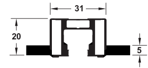
Lateral frame profile No.52 h เฟรมด้านข้างเบอร์ 52 h
