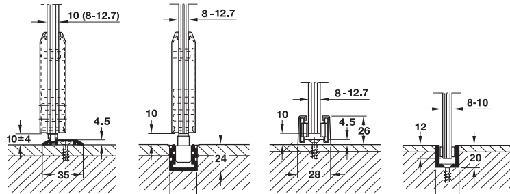
Built-in version 1 โค้ดล่าง รูปแบบที่ 1 Built-in version 2 โค้ดล่าง รูปแบบที่ 2 Built-in version 3 โค้ดล่าง รูปแบบที่ 3 Built-in version 4 โค้ดล่าง รูปแบบที่ 4
