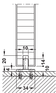
Without guide track แบบไม่มีรางล่าง
