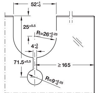
Required glass cut-outs กรุณาคัดกระจกตามรูปแบบที่กำหนดเท่านั้น
