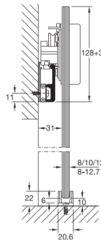
Wall mounting Model A1, E1 ติดตั้งบนผนัง รูปแบบ A1, E1
