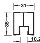
Lateral frame profile 20 เฟรมด้านข้างเบอร์ 20
