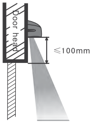
Surface mounted การติดตั้งแบบติดลอย
