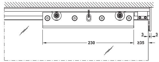
Section trolley hanger 80–120 kg ระยะการติดตั้งสำหรับแขนลูกล้อ 80-120 กก.
