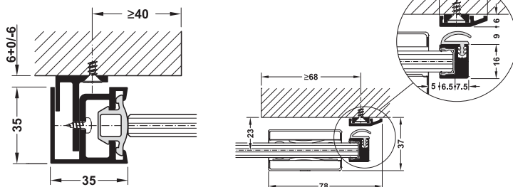
Wall profile set include rubber seal การติดตั้งรางซีลที่ผนัง
