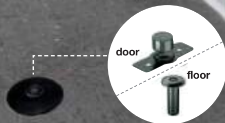
938.70.003 Magnetic door stop Polycarbonate Black กันชนประตูแบบมีแม่เหล็ก โพลีคาบอเนต สีดำ
