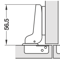
Half overlay แบบกลางขอบ
