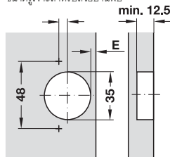
Drilling dimension for cup fixing ขนาดรูเจาะสำหรับถ้วยบานพับ
