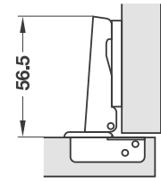
Full overlay แบบทับขอบ
