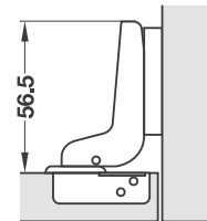
Inset แบบในขอบ
