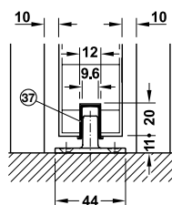
With guide track แบบติดตั้งรางใต้บาน
