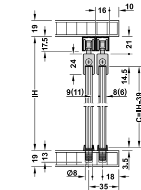
For screw fixing ติดตั้งรางบนแบบติดลอยด้วยสลัก
