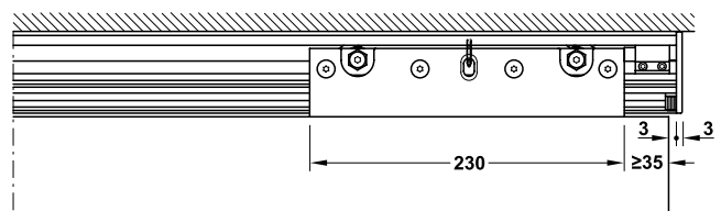
Section trolley hanger 80E/120E with soft and self closing mechanism ระยะการติดตั้งลูกล้อพร้อมระบบปิดนุ่มนวล รุ่น 80E/120E
