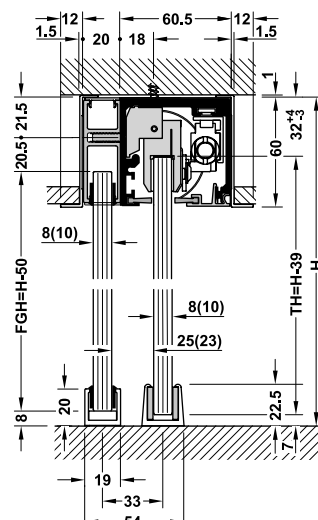
With fixed element, with supporting bracket มีบานติดตาย พร้อมโครงรับฝ้า
