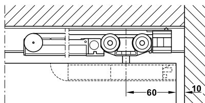
With soft and self closing mechanism มีอุปกรณ์ปิดแบบนุ่มนวล
