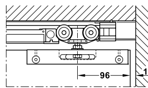
With soft and self closing mechanism มีอุปกรณ์ปิดแบบนุ่มนวล
