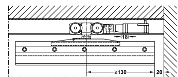
Track stopper with magnetic pull อุปกรณ์หยุดบานผลักเพื่อเปิดแบบมีแม่เหล็ก
