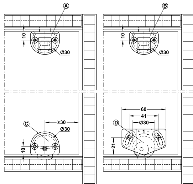
Running gear without height adjustment ลูกกลิ้งแบบไม่มีตัวปรับความสูงบานประตู
