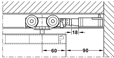
With Push-to-Open with magnetic pull มีอุปกรณ์หยุดบานผลักเพื่อเปิดแบบแม่เหล็ก
