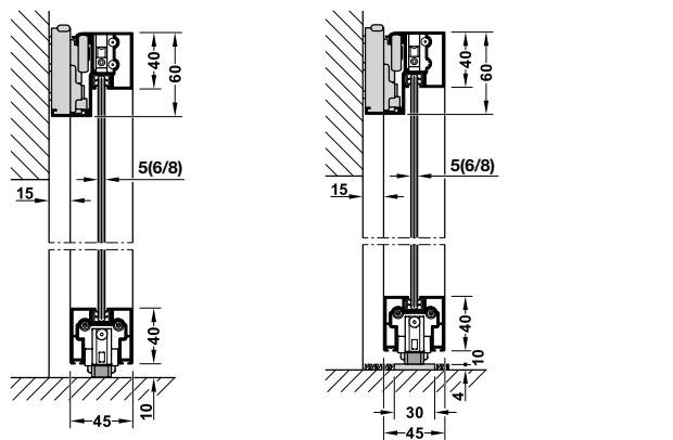
Floor guidance on hard floors สำหรับติดตั้งพื้นทั่วไป
