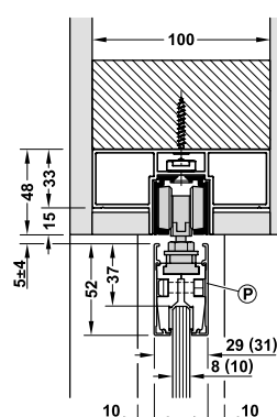
With SLIDO D-Line11 L รุ่น With SLIDO D-Line11 L
