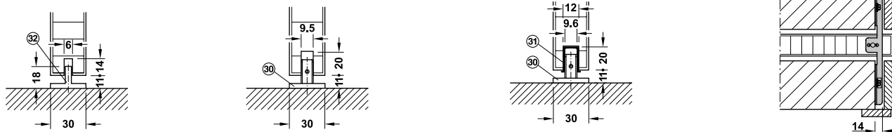
Standard floor guide กันแกว่งมาตรฐาน
