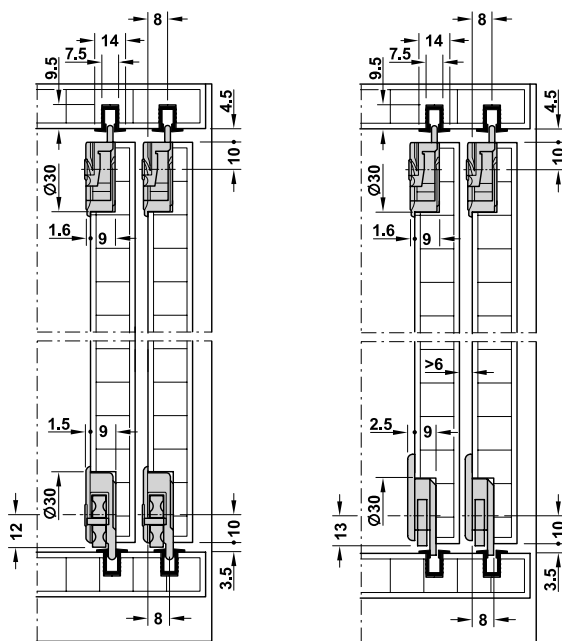
Running gear without height adjustment ลูกกลิ้งแบบไม่มีตัวปรับความสูงบานประตู
