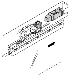
Track stopper อุปกรณ์หยุดบานผลักเพื่อเปิด
