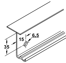
With stopper for rear door สำหรับตัวหยุดประตูบานใน
