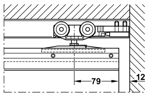
With track buffer with retaining spring มีอุปกรณ์หยุดบานพร้อมส่วนยึดลูกกลิ้งแบบยึดหยุ่น
