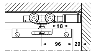
With Push-to-Open มีอุปกรณ์หยุดบานผลักเพื่อเปิด
