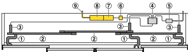
For 4 doors, centre door synchronized running สำหรับ 4 บานประตู, บานประตูคู่กลาง เปิด-ปิด พร้อมกัน
