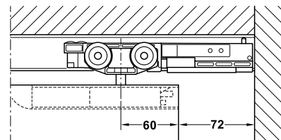
With shock absorber with retaining spring มีอุปกรณ์หยุดบานแบบนุ่มนวลพร้อมสปริง
