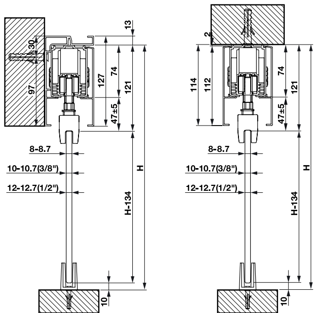
Wall installation with glass panel ติดตั้งบนผนัง สำหรับประตูบานกระจก
