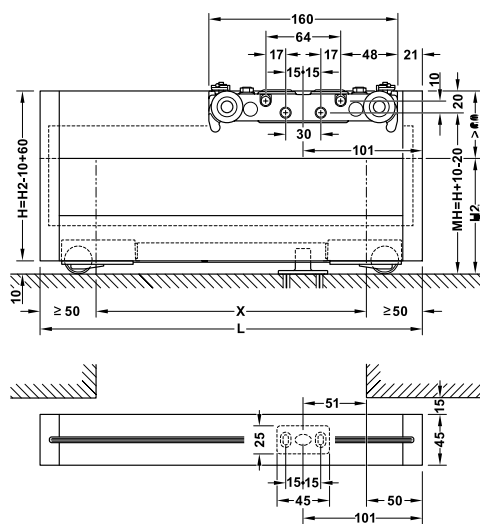
Floor guidance on hard floors สำหรับติดตั้งพื้นทั่วไป
