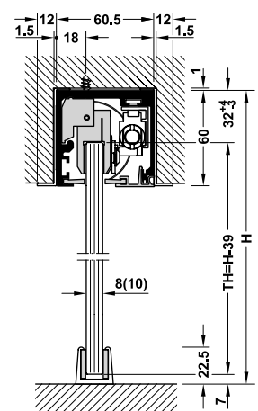
With fixed element, with supporting bracket มีบานติดตาย พร้อมโครงรับฝ้า
