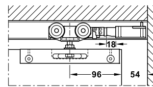
With Push-to-Open with magnetic pull มีอุปกรณ์หยุดบานผลักเพื่อเปิดแบบแม่เหล็ก
