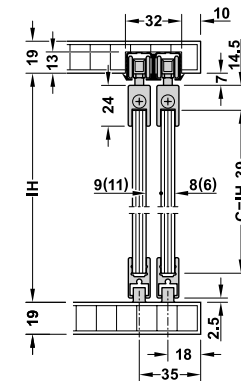
For groove mounting ติดตั้งรางบนแบบฝัง
