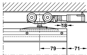
With Push-to-Open with magnetic pull มีอุปกรณ์หยุดบานผลักเพื่อเปิดแบบแม่เหล็ก
