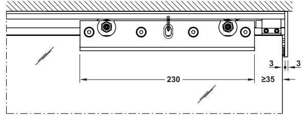
Section trolley hanger 80F/120F without soft- and self-closing mechanism ระยะการติดตั้งลูกล้อไม่มีระบบปิดนุ่มนวล รุ่น 80F/120F
