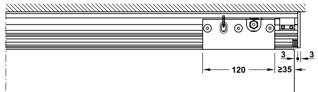
Section trolley hanger 50E without soft and self closing mechanism ระยะการติดตั้งลูกล้อไม่มีระบบปิดนุ่มนวล รุ่น 50E
