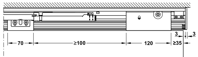
Section trolley hanger 50E with soft and self closing mechanism ระยะการติดตั้งลูกล้อพร้อมระบบปิดนุ่มนวล รุ่น 50E
