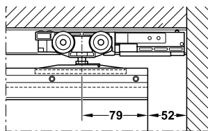
With shock absorber with retaining spring มีอุปกรณ์หยุดบานแบบนุ่มนวลพร้อมสปริง
