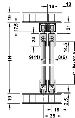
For screw fixing ติดตั้งรางบนแบบติดลอยด้วยสลัก
