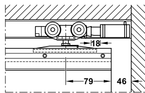
With Push-to-Open มีอุปกรณ์หยุดบานผลักเพื่อเปิด
