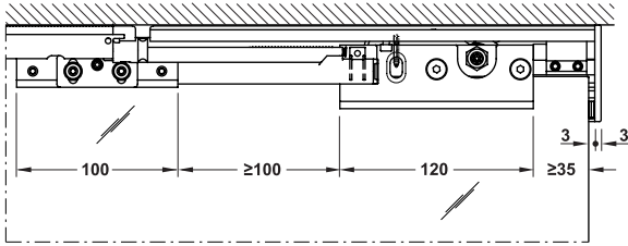
Section trolley hanger 50F with soft- and self-closing mechanism ระยะการติดตั้งลูกล้อพร้อมระบบปิดนุ่มนวล รุ่น 50F
