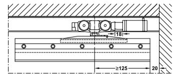
Track stopper อุปกรณ์หยุดบานผลักเพื่อเปิด
