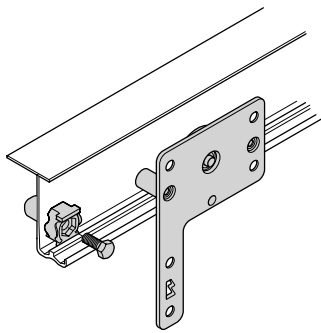
Running gear, rear door การติดตั้งลูกกล้อประตูบานใน
