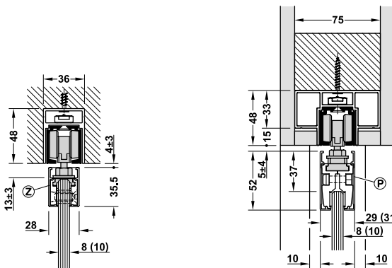
With SLIDO D-Line11 J รุ่น SLIDO D-Line11 J
