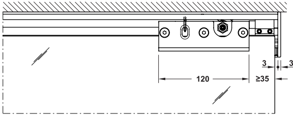
Section trolley hanger 50F without soft- and self-closing mechanism ระยะการติดตั้งลูกล้อไม่มีระบบปิดนุ่มนวล รุ่น 50F
