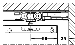
With shock absorber with retaining spring มีอุปกรณ์หยุดบานแบบนุ่มนวลพร้อมสปริง
