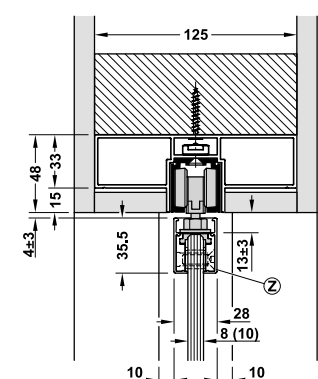
With SLIDO D-Line11 J รุ่น With SLIDO D-Line11 J
