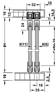
For groove mounting ติดตั้งรางบนแบบฝัง
