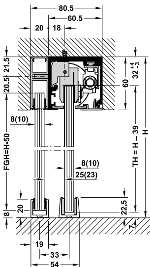
With fixed element มีบานติดตาย
