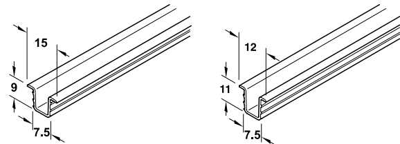
Aluminium รางอะลูมิเนียม
