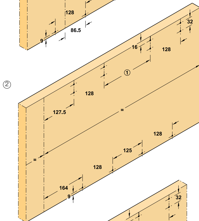
② For 3 doors, left and right (mirror-inverted) แบบเจาะสำหรับตู้ 3 บาน, บานซ้าย และบานขวา (ด้านตรงข้าม)
