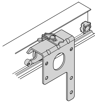
Running gear, front door การติดตั้งลูกกล้อประตูบานนอก
