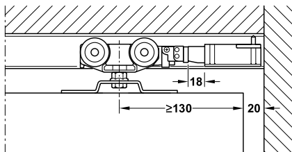
Track stopper with magnetic pull อุปกรณ์ผลักเพื่อเปิดสำหรับหยุดบาน
