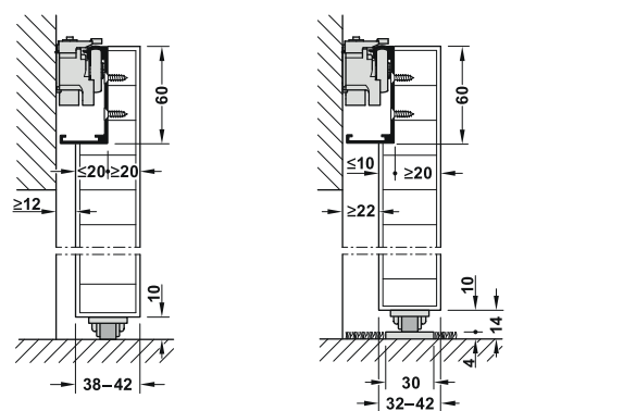
Floor guide on hard floor การติดตั้งบนพื้นแข็ง
