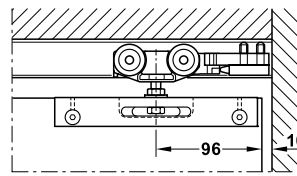
With track buffer with retaining spring มีอุปกรณ์หยุดบานพร้อมส่วนยึดลูกกลิ้งแบบยึดหยุ่น
