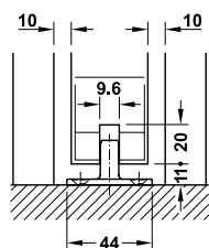
Without guide track แบบไม่มีรางใต้บาน
