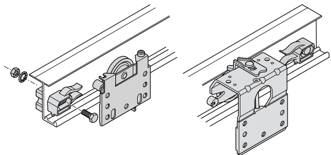
Running gear, rear door การติดตั้งลูกกลิ้งประตูบานใน
