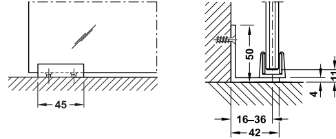
Section floor guide ระยะการติดตั้งสำหรับอุปกรณ์กันแกว่ง
