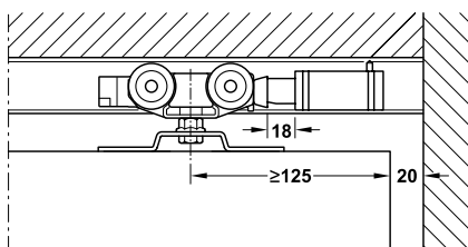
Track stopper อุปกรณ์หยุดบานผลักเพื่อเปิด
