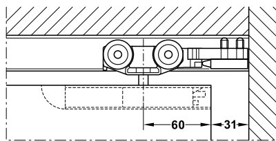
With track buffer with retaining spring มีอุปกรณ์หยุดบานพร้อมส่วนยึดลูกกลิ้งแบบยึดหยุ่น
