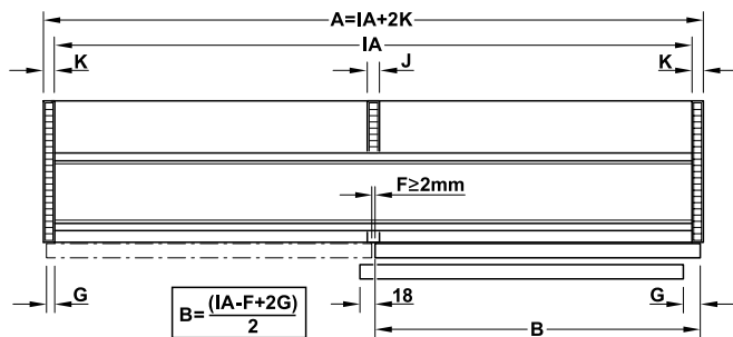
2-leaf version สำหรับ 2 บานประตู
