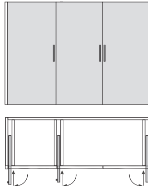
Doors closing against base and top section บานทับขอบ บน-ล่าง
