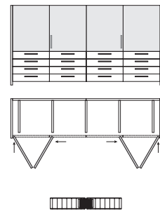
Optional: Door centring with magnetic centring elements อุปกรณ์เสริม: ประตูตู้ปิดกลางด้วยกลไกแม่เหล็ก
