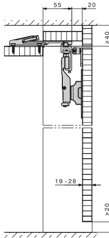
Optional: Door centring with magnetic centring elements อุปกรณ์เสริม: ประตูตู้ปิดกลางด้วยกลไกแม่เหล็ก
