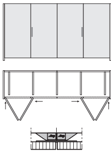
Optional: Door centring with leading ramp อุปกรณ์เสริม: ประตูตู้ปิดกลางด้วยไกด์ประตู
