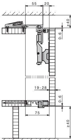
Optional: Door centring with leading ramp อุปกรณ์เสริม: ประตูตู้ปิดกลางด้วยไกด์ประตู
