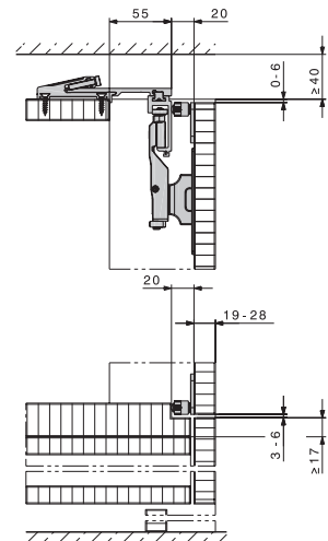
Optional: Door centring with magnetic centring elements อุปกรณ์เสริม: ประตูตู้ปิดกลางด้วยกลไกแม่เหล็ก
