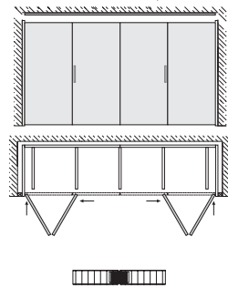
Optional: Door centring with magnetic centring elements อุปกรณ์เสริม: ประตูตู้ปิดกลางด้วยกลไกแม่เหล็ก
