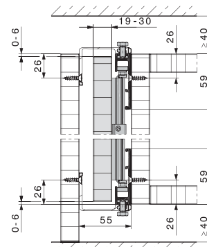
HAWA-Concepta 25 30 with connector 55 mm HAWA-Concepta 25 30 ติดด้วยแผ่นยึดขอบ ขนาด 55 มม.
