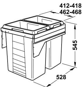
Two compartment waste bin ถังขยะแบบ 2 ช่อง
